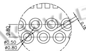
DETAIL I 2 : 1
